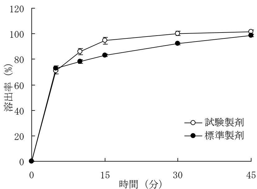
図3 カルジール細粒20%の溶出試験結果 (pH6.8, 50rpm)
