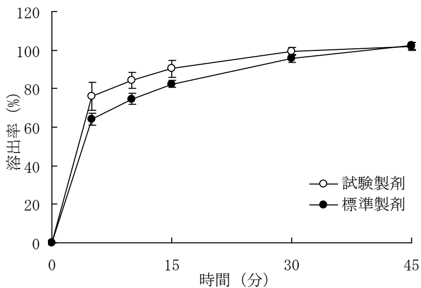
図1 カルジール細粒 20%の溶出試験結果 (pH1.2, 50rpm)
