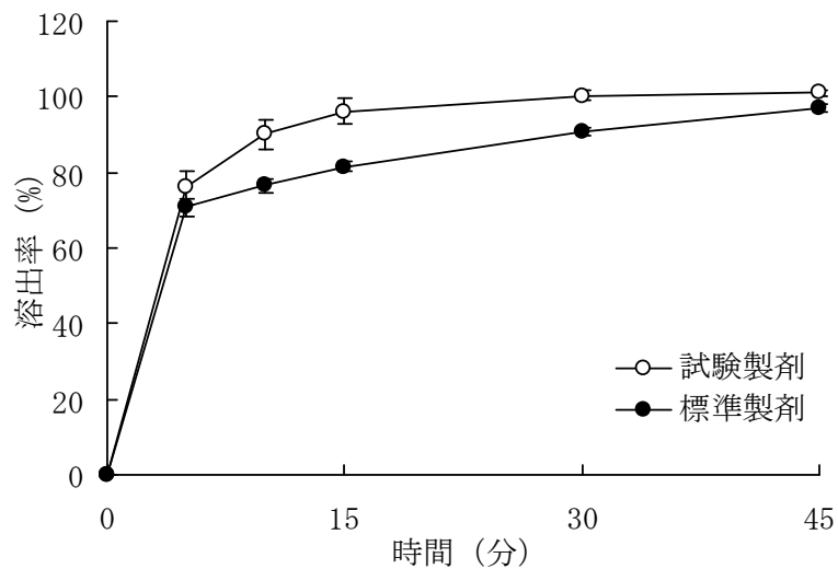
図 2 溶出曲線 (pH5.5、50rpm)
