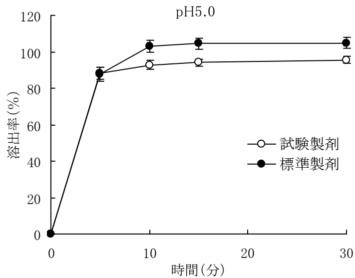
図2 セフポドキシムプロキセチルドライシロップ5%「タイヨー」 の溶出試験結果 (pH5.0, 50rpm)
