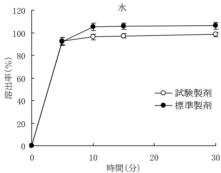
図4 セフポドキシムプロキセチルドライシロップ5%「タイヨー」 の溶出試験結果（水，50rpm）
