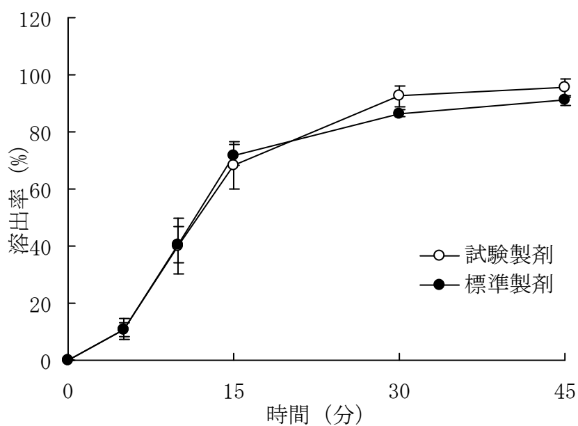
図4 ナフトジール錠2の溶出試験結果（水，50rpm）
