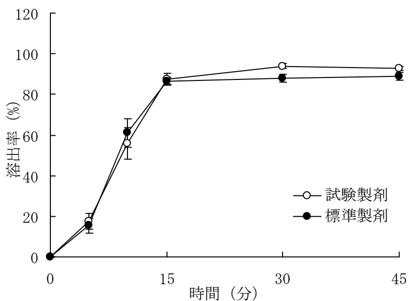
図5 ナフトジール錠2の溶出試験結果 (pH6.8, 100rpm)
