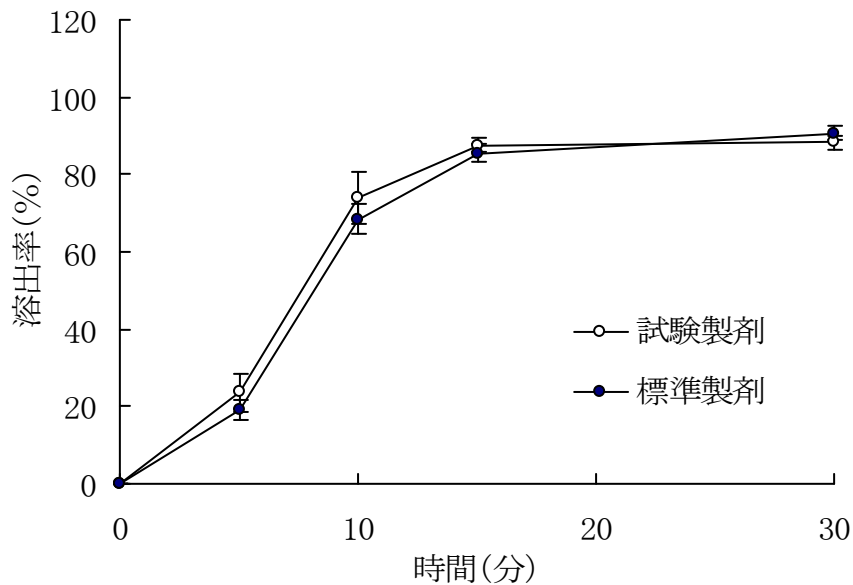
図4 ナフトジール錠4の溶出試験結果(水, 50rpm)
