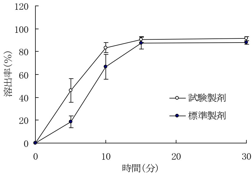
図1 ナフトジール錠4の溶出試験結果 (pH1.2, 50rpm)
