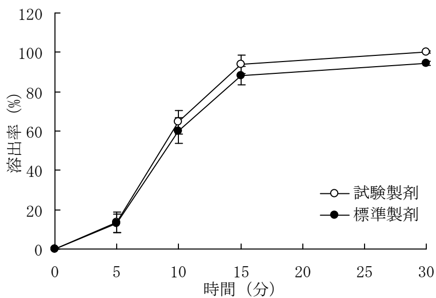
図2 ニセルゴリン錠5mg「タイヨー」の溶出試験結果 (pH4.0, 50rpm)
