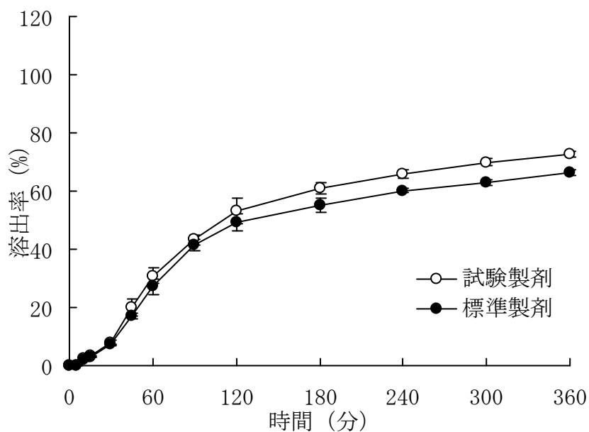
図4 ニセルゴリン錠 5mg 「タイヨー」の溶出試験結果 (水, 50rpm)
