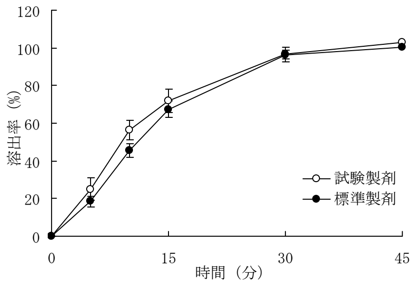
図1 マニジピン塩酸塩錠 20mg 「タイヨー」の溶出試験結果 (pH1.2, 50rpm)
