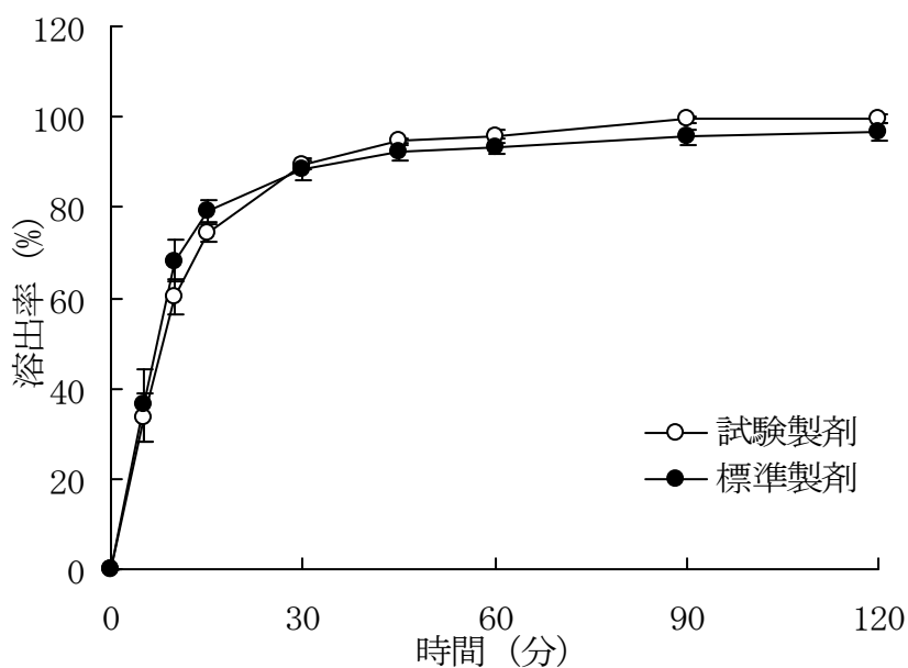
図3 メロキシカム錠5mg「タイヨー」の溶出試験結果 (pH6.8, 50rpm)
