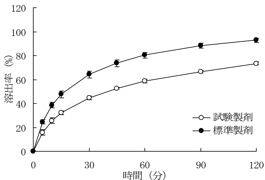
図5 メロキシカム錠5mg「タイヨー」の溶出試験結果 (pH5.5, 100rpm)
