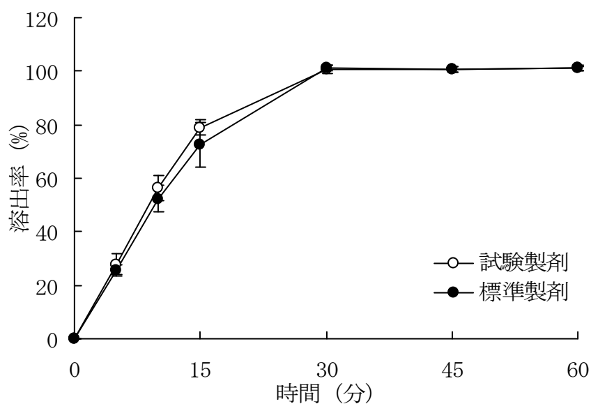
図2 メトプリック錠 20mg の溶出試験結果 (pH4.0, 50rpm)
