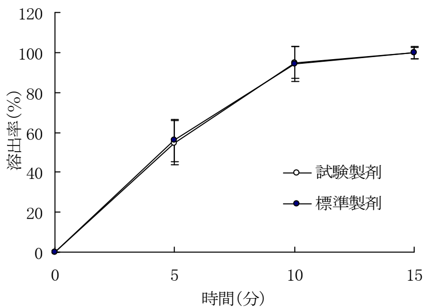
図1 ミルナシプラン塩酸塩錠 15mg 「タイヨー」の溶出試験結果 (pH1.2, 50rpm)
