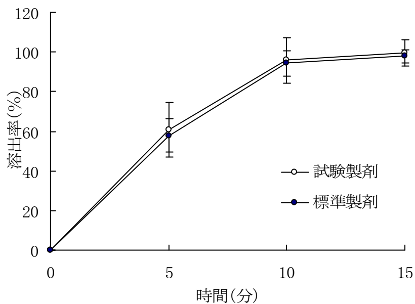
図2 ミルナシプラン塩酸塩錠 15mg 「タイヨー」の溶出試験結果 (pH3.0, 50rpm)
