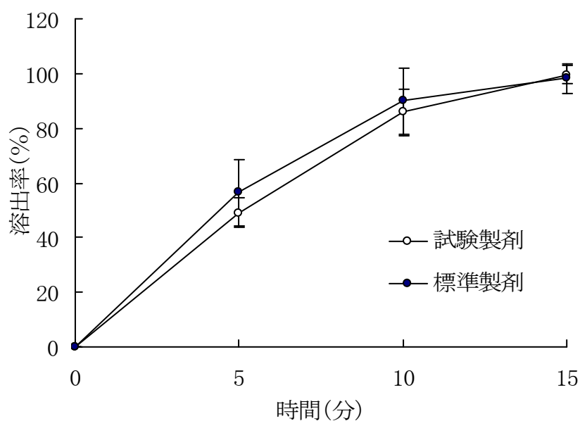
図1 ミルナシプラン塩酸塩錠 25mg 「タイヨー」の溶出試験結果 (pH1.2, 50rpm)
