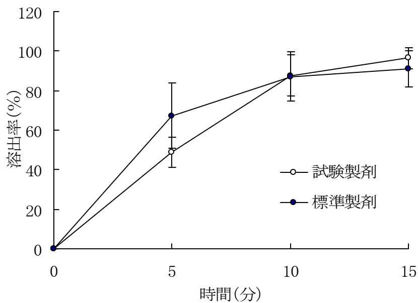
図3 ミルナシプラン塩酸塩錠 25mg「タイヨー」の溶出試験結果 (pH6.8, 50rpm)
