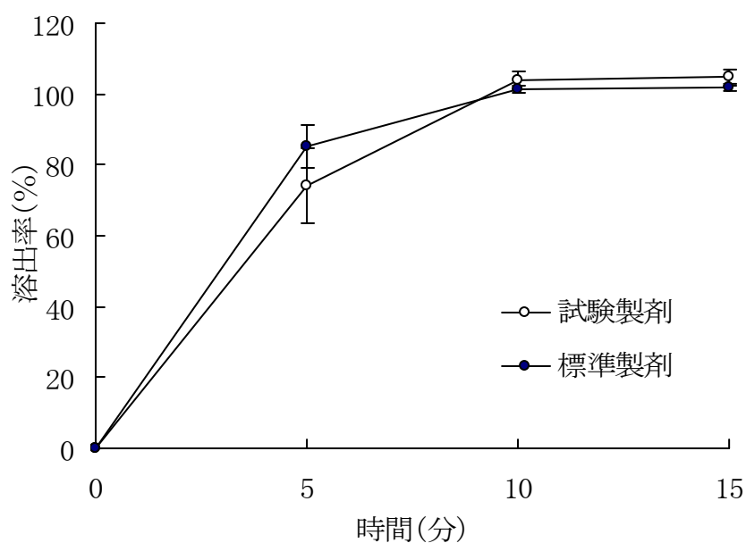
図2 ミルナシプラン塩酸塩錠 25mg「タイヨー」の溶出試験結果 (pH5.0, 50rpm)
