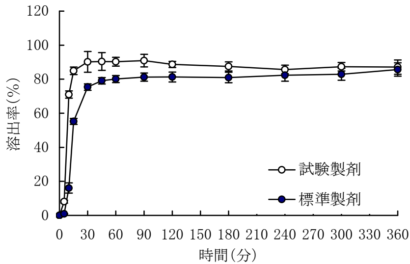
図4 ランソプラゾール OD錠 30mg 「タイヨー」の溶出試験結果 (pH6.0, 100rpm)
